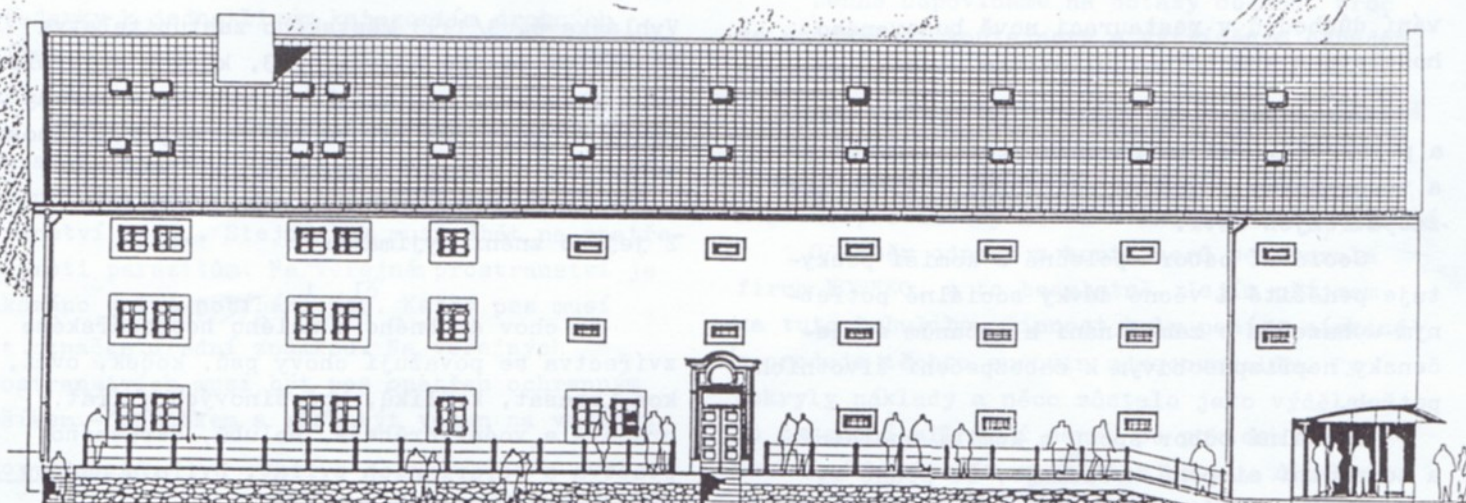
POHLED BOČNÍ Z HUSOVA NÁMĚSTÍ – 1:100
